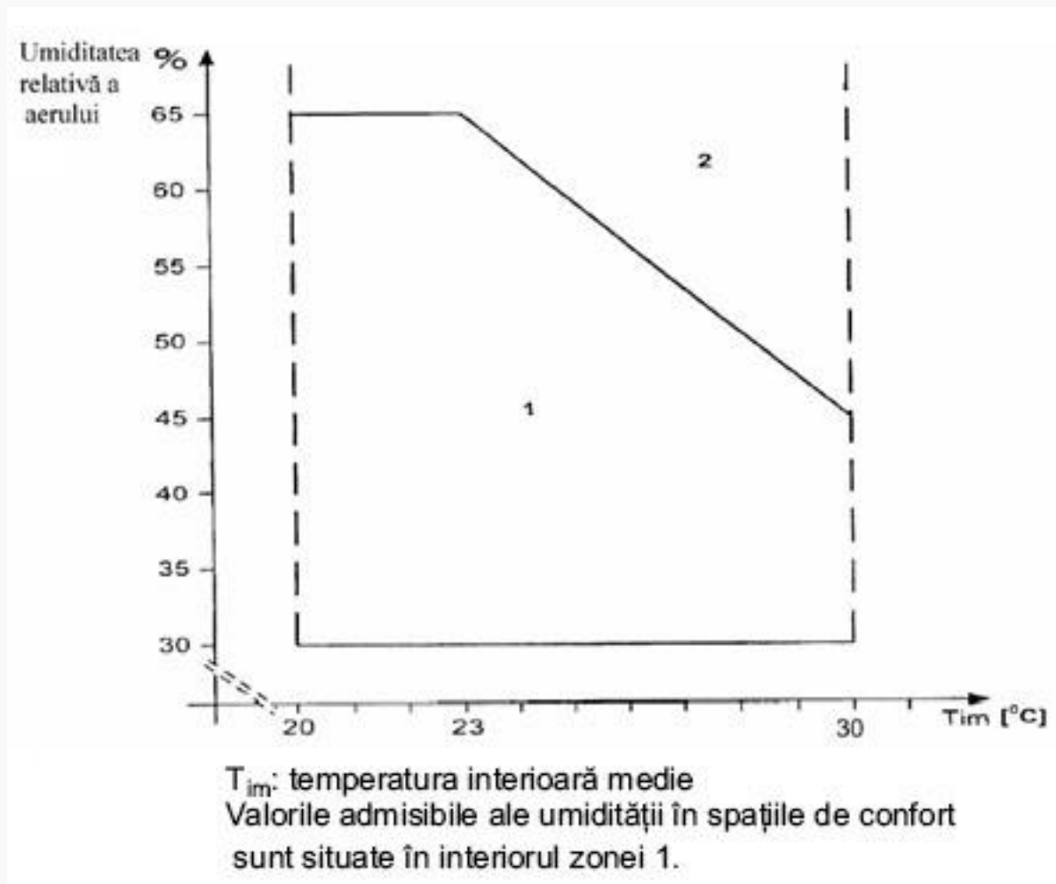
Figura nr. 6*) - Umiditatea relativă a aerului în spațiile de confort
