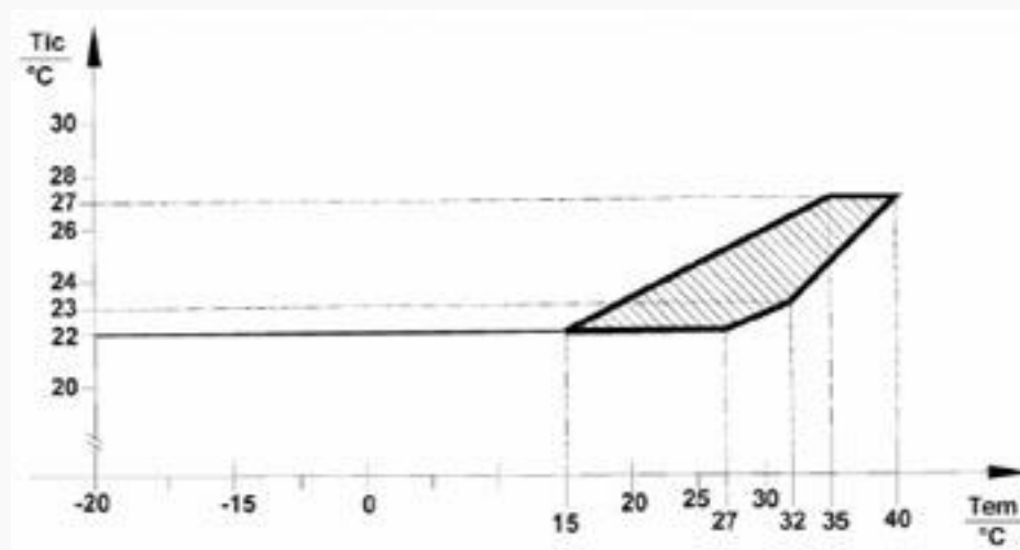
Figura nr. 4*) - Curba de reglaj pentru temperatura interioară prescrisă
