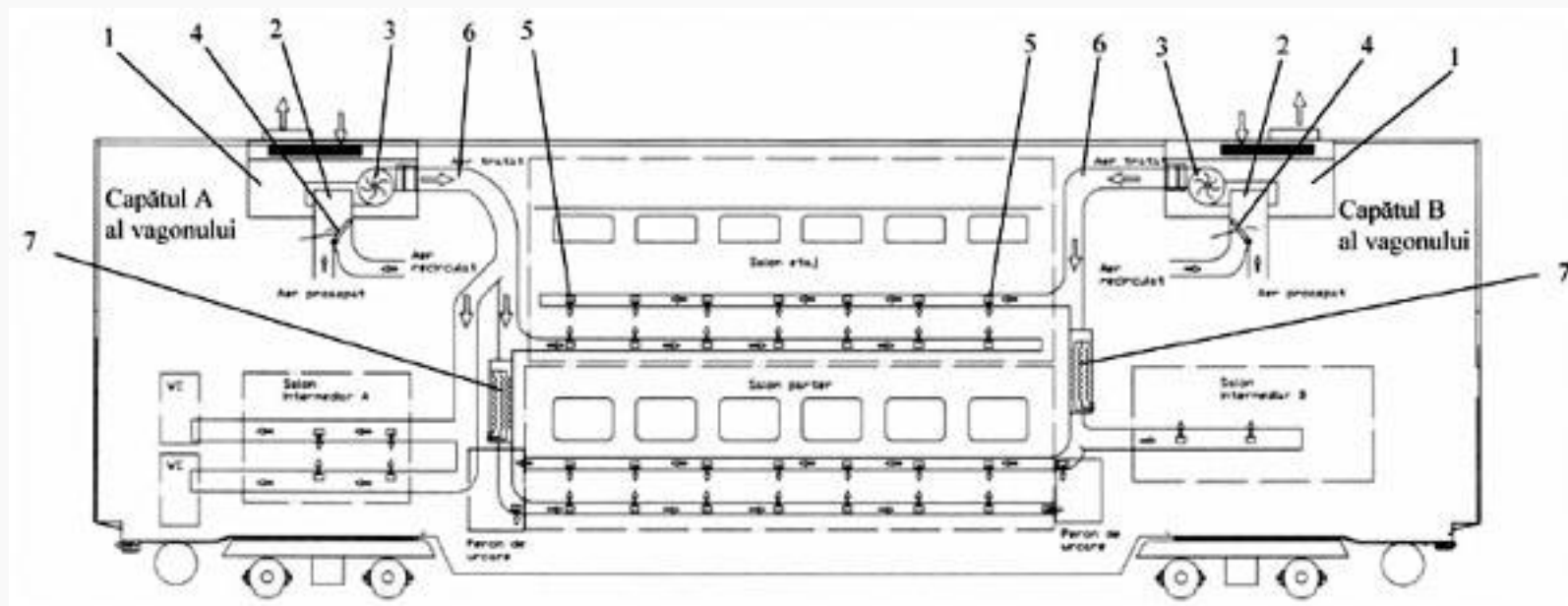
Figura nr. 3*) - Exemplu de componență a instalației de ventilație/încălzire/climatizare aer pentru un vagon cu două niveluri
